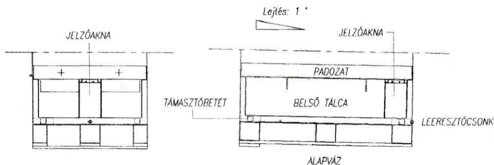
02. ábra Alsó tálcarendszer metszeti rajza
